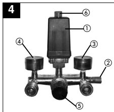
6 Prekidač
